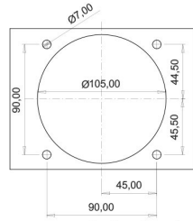
PUNCH DELİK ÖLÇÜLERİ
