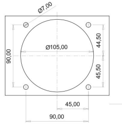
PUNCH DELİK ÖLÇÜLERİ
