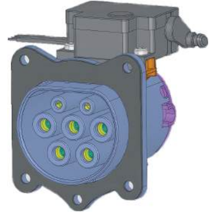
Her iki tipe uyumlu tek gövde tasarımı.
